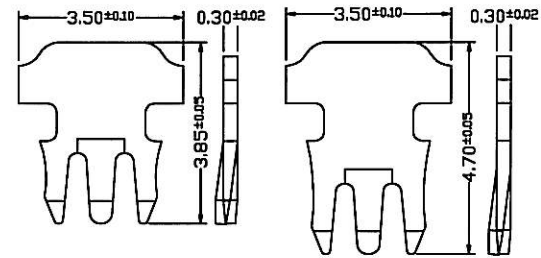
コンタクトブレード形状
