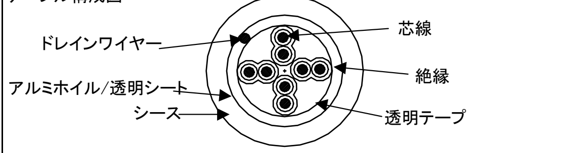
ケーブル構成図
